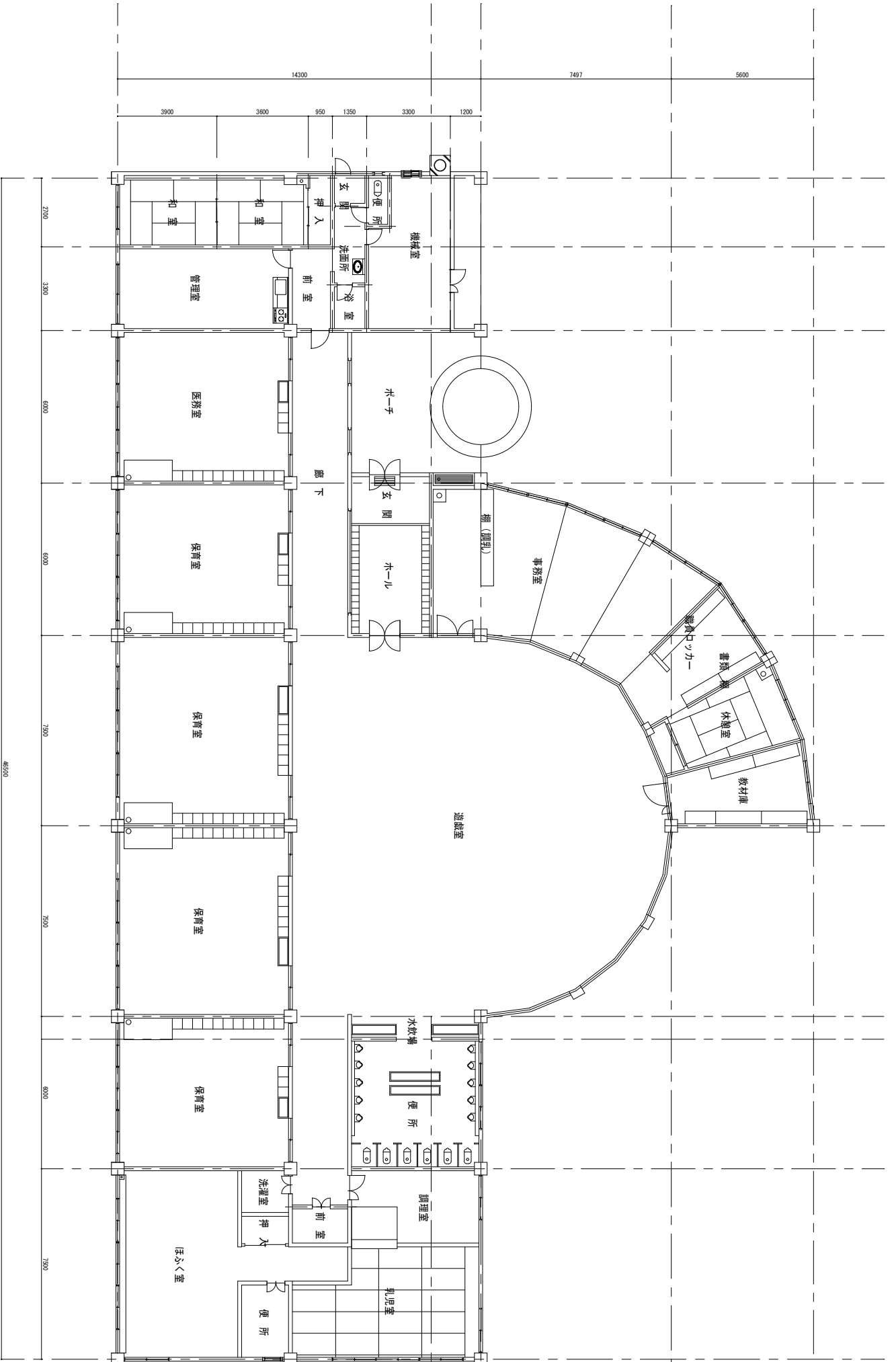
栄町保育所 平面図
