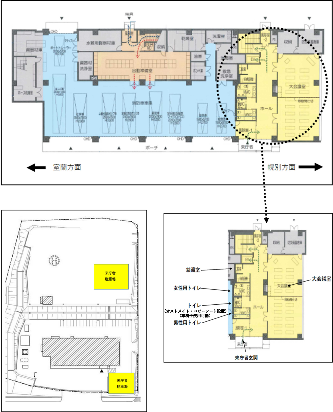
登別市消防庁舎 1 階平面図（大会議室位置図）
