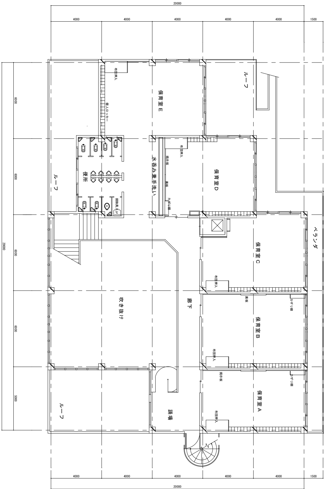
梶別東保育所 2階平面図
